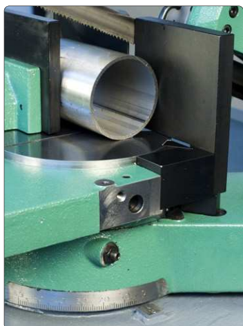
(*) Spalle morsa arretrabili per ottenere la massima capacità di taglio (340 x 180 mm). Scala graduata incisa di facile ed agevole lettura
