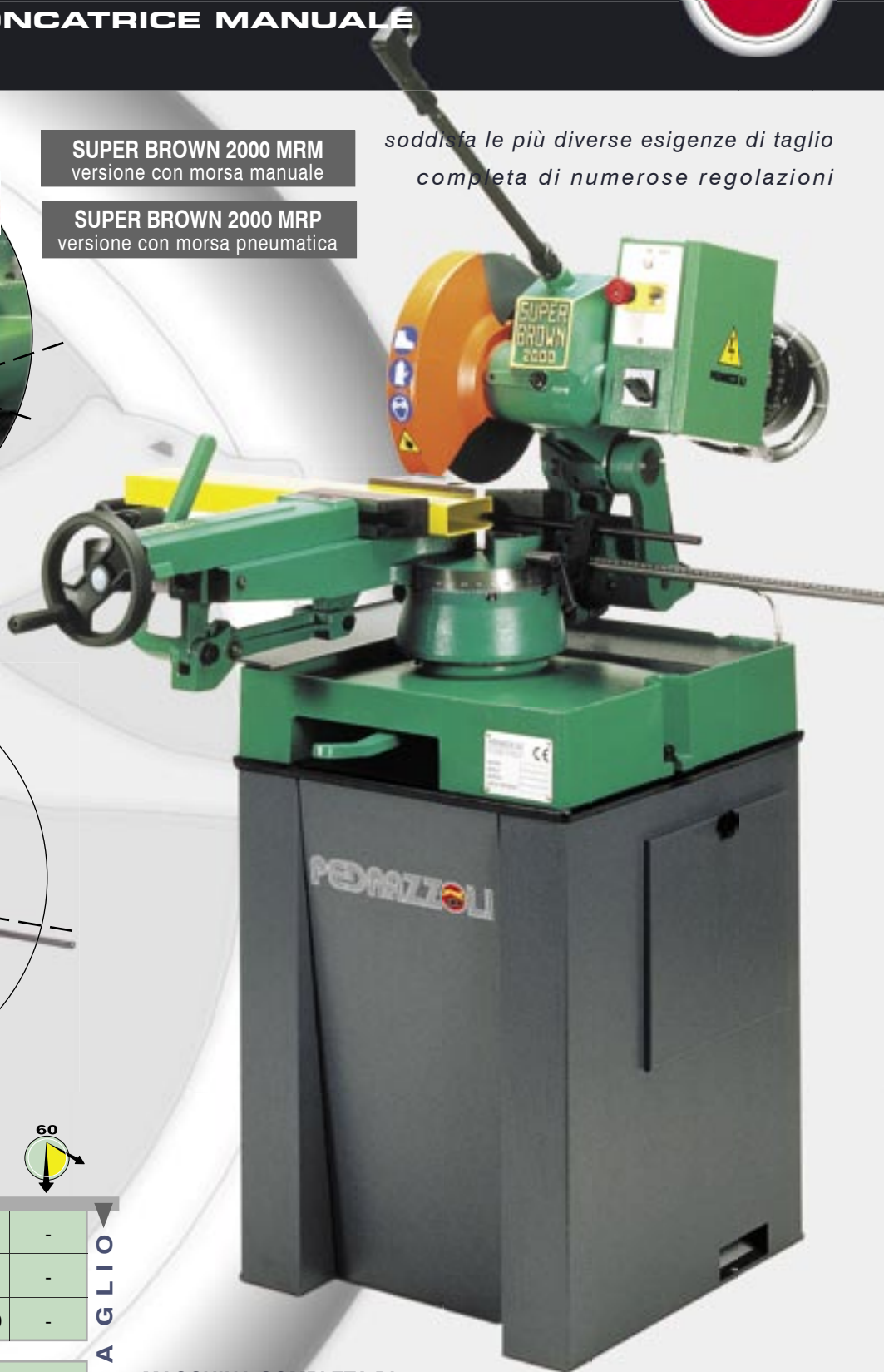
Gruppo di movimentazione laterale testa per tagli a 45° sulla verticale a sinistra e tagli longitudinali.
