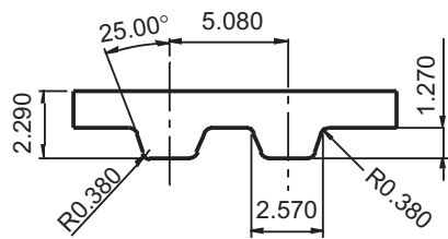
Fig.2 Passo 5.080mm (XL)
