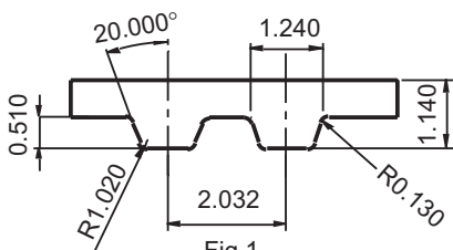
Fig.1 Passo 2.032mm (MXL)
